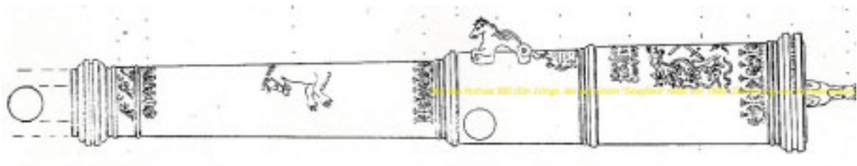
Zeichnung des Rohres 380 von Andreas Herold im Armeemuseum Stockholm, Zeichnung: Königliches Armeemuseum Stockholm
