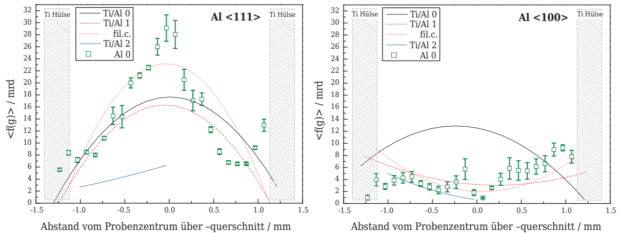
Abbildung 4.12: Gradient der Al \langle 111 \rangle + \langle 100 \rangle -Doppelfasertextur des Al 0 Drahtes im Vergleich zu jenem der Ti/Al 0-2 Drähte (vgl. Abbildung 4.10 ): Gradient der integrierten Fasermaximalwerte
