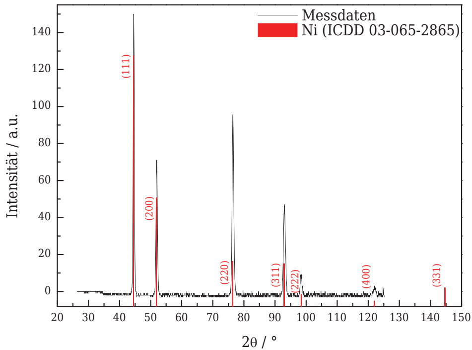
Abbildung 4.21: XRDg des UFK ED Ni-5at.%Fe, gemessen mittels des XRμD 2 -Systems; nach [197]
