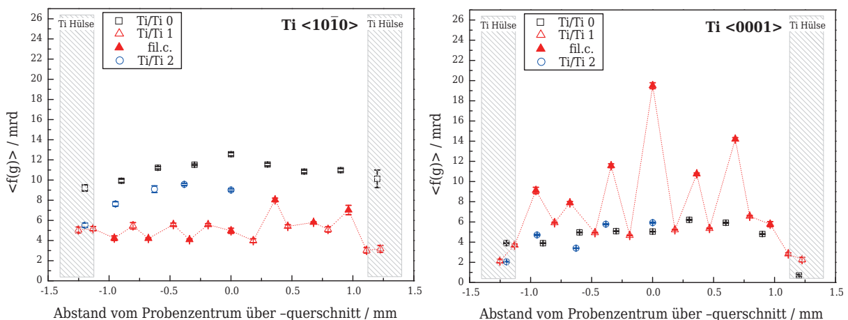
Abbildung 4.16: Gradient der Ti Textur der Ti/Ti 0-2 Drähte: Gradient der integrierten Fasertexturen \langle 10\bar{1}0 \rangle und \langle 0001 \rangle
