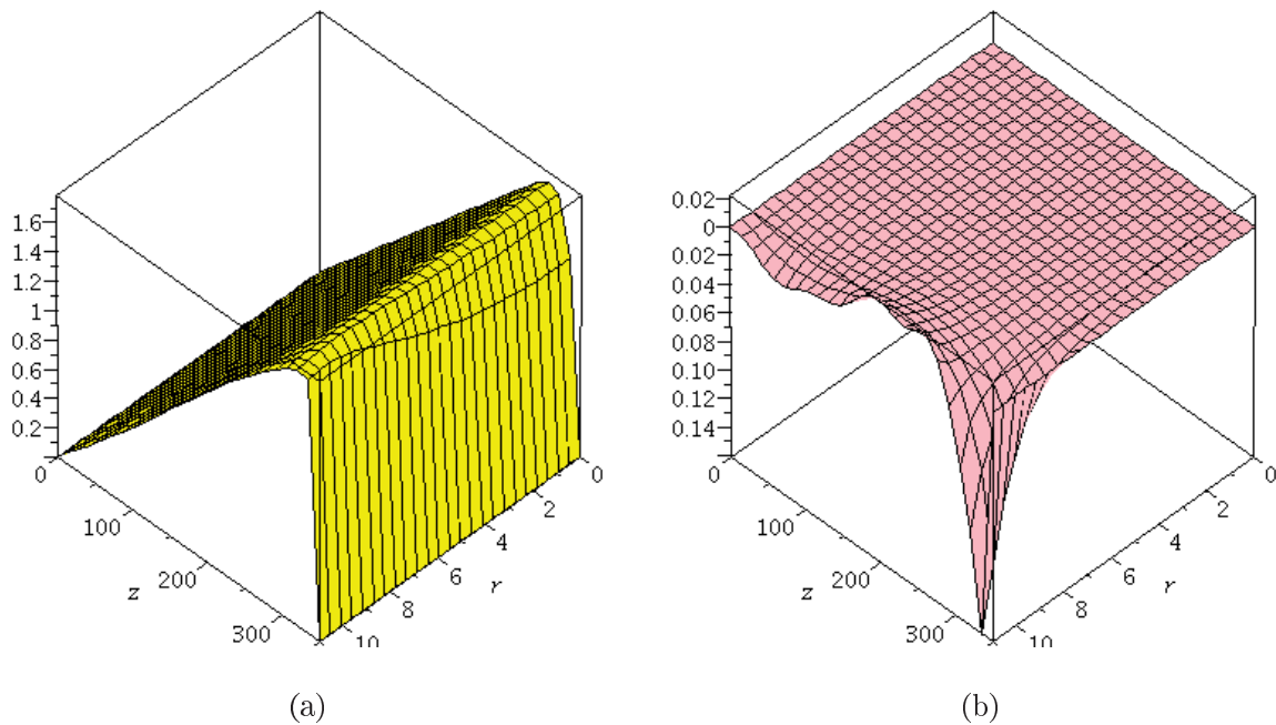
Abbildung 4.49: Partiaillösung \hat{u}_{z,I} : (a) Reihenapproximation mit 50 Summanden, (b) Variation der nächsten 150 Summanden
