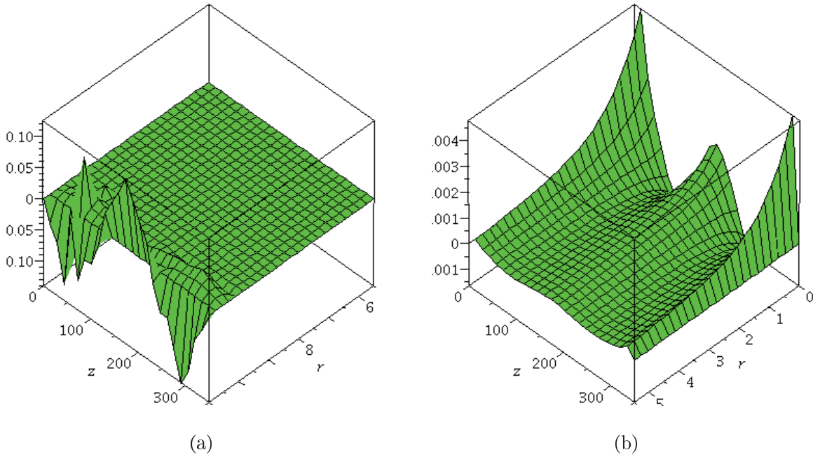
Abbildung 4.52: Partillösung u_{z,III} : Variation der nächsten 25 Summanden in der Reihenapproximation für (a) r \in [r_a/2, r_a] bzw. (b) r \in [0, r_a/2]
