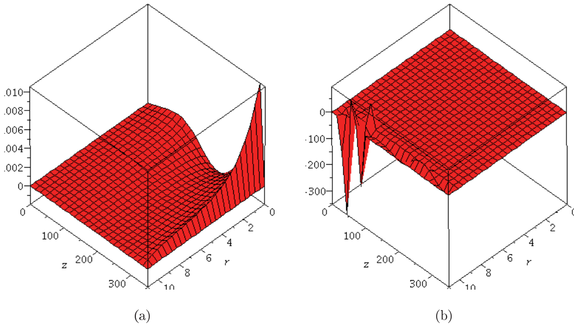
Abbildung 4.54: Partiaillösung \tilde{u}_z - u_{z,III} von \ddot{u}_z(r, z) : Variation der nächsten (a) 50 Summanden, bzw. (b) 150 Summanden
