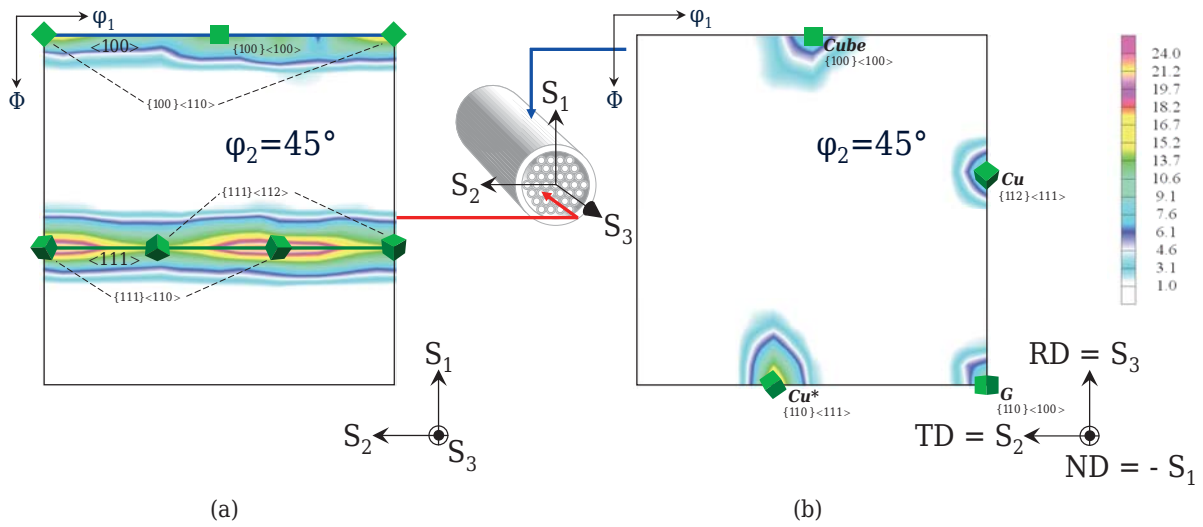
Abbildung 4.7: Schlüsselfigur zur Identifikation der Al Texturkomponenten inkl. der Lagebeziehung der beiden Referenzsysteme: (a) ASB PKS S und (b) PKS ebener Verformung; nach [8]
