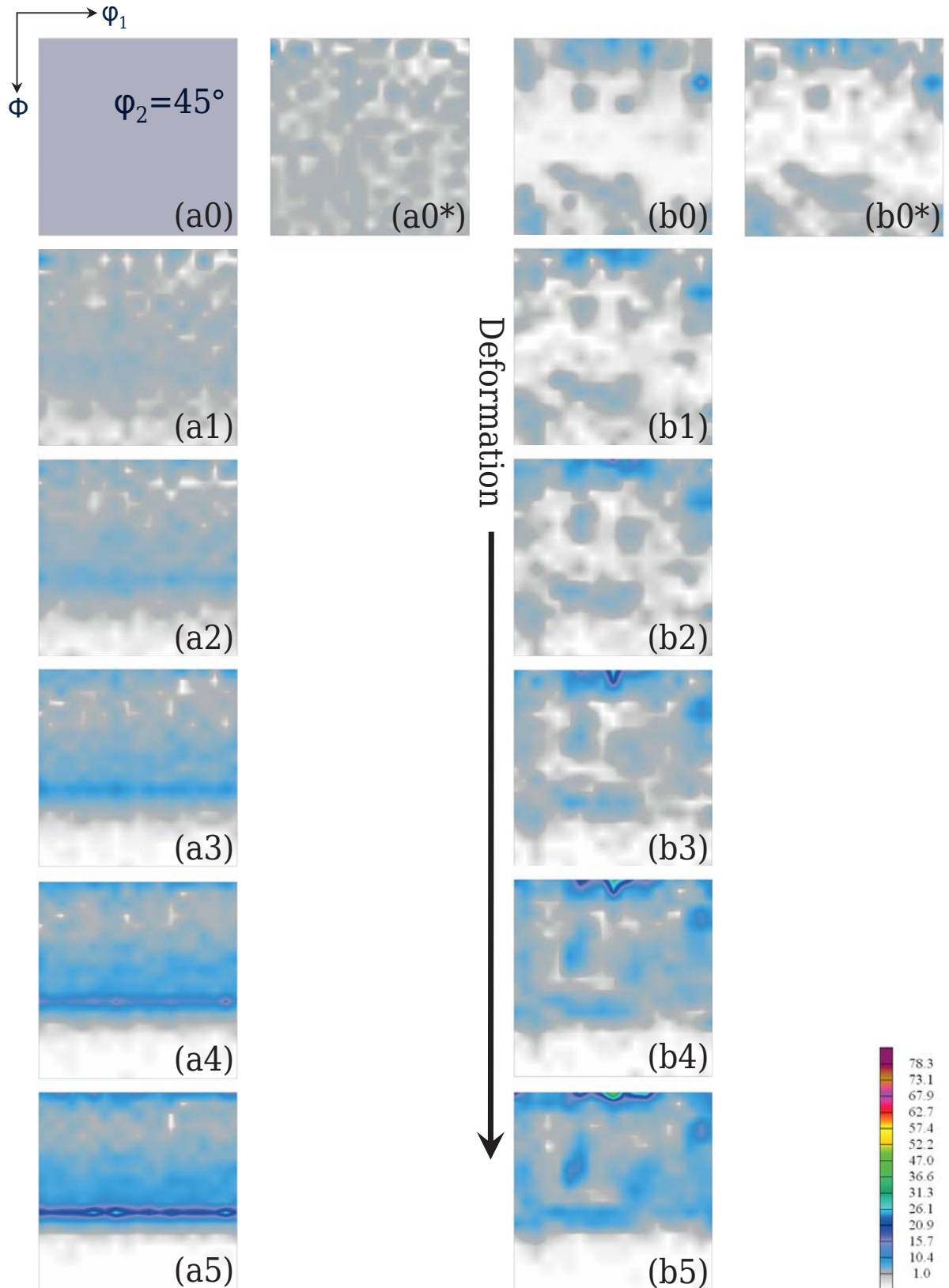
Abbildung 4.39: VPSC Textursimulationsergebnis für Al in Ti/Al O (rechts) sowie einer zunächst regellosen Textur (links) im Vergleich nach (4.17): Texturevolution in 0.0883 Dehnungsincrementen (bei a = -0.6 , b = -0.4 ); Fortsetzung in Abbildung 4.40
