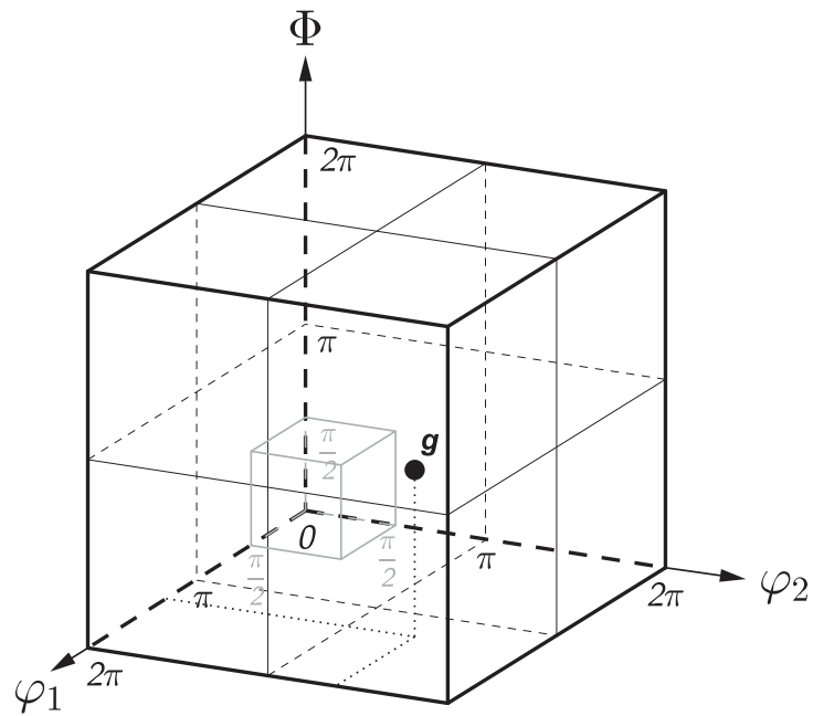
Abbildung 2.11: Zur im 3D EULERRaum, anhand der drei EULERwinkel \varphi_1 , \Phi und \varphi_2 definierten kristallografischen Orientierung g ; nach [3]
