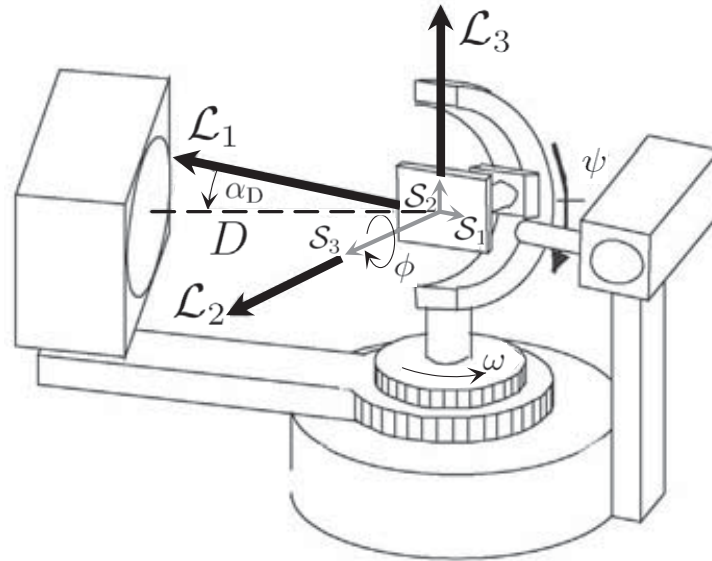
Abbildung 2.8: Diffraktometerkonfiguration des XRμD 2 Messsystems; nach [3]
