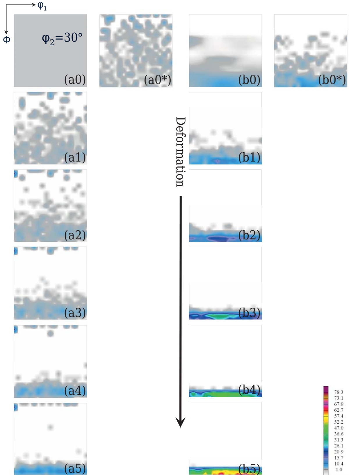
Abbildung 4.44: VPSC Textursimulationsergebnis für Ti in Ti/Al 0 (rechts) sowie einer zunächst regellosen Textur (links) im Vergleich nach (4.19): Texturevolution in 0.0883 Dehnungsincrementen (bei a = -0.5 = b , d = 0.0 , e = 0.2 ); Fortsetzung in Abbildung 4.45
