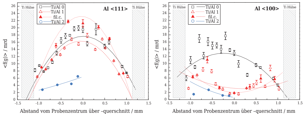
Abbildung 4.10: Gradient der Al \langle 111 \rangle + \langle 100 \rangle -Doppelfasertextur der Ti/Al 0-2 Drähte: Gradient der integrierten Fasermaximalwerte
