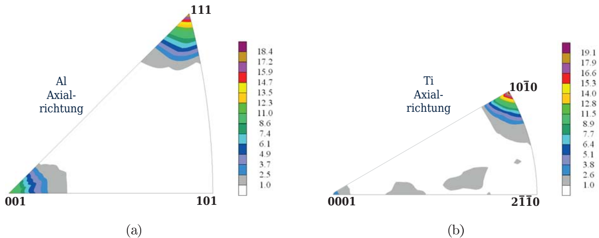
Abbildung 4.6: INVPF der Lokaltextrur des Ti/Al 0 Drahtes (Drahtachse bei Messung entsprechend Abbildung 4.5 ): (a) Al, (b) Ti; nach [8]
