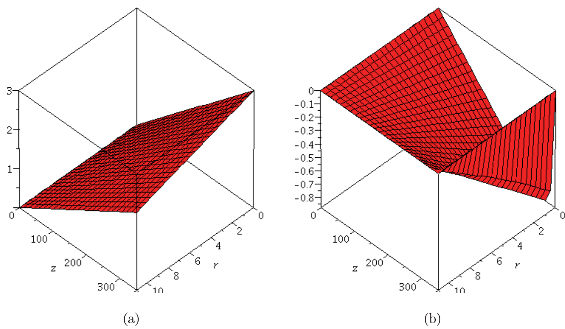
Abbildung 4.53: Partillösungen von \ddot{u}_z(r, z) : (a) bilineare Funktion \ddot{u}_{z,b} , (b) zusätzliche Partillösung \tilde{u}_z - u_{z,III} nach (4.54)
