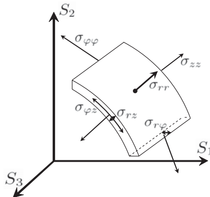
Abbildung 4.29: Zylindrische Spannungstensoranteile am Ausschnitt einer Probenhülse im Bezug zum Probenkoordinatensystem \mathcal{S} [7]
