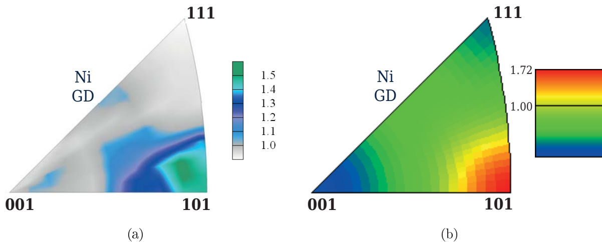
Abbildung 4.23: Textur des UFK ED Ni-5at.%Fe: INVPF in GD aus (a) der XRµD 2 -ta bzw. aus (b) EBSD Messungen
