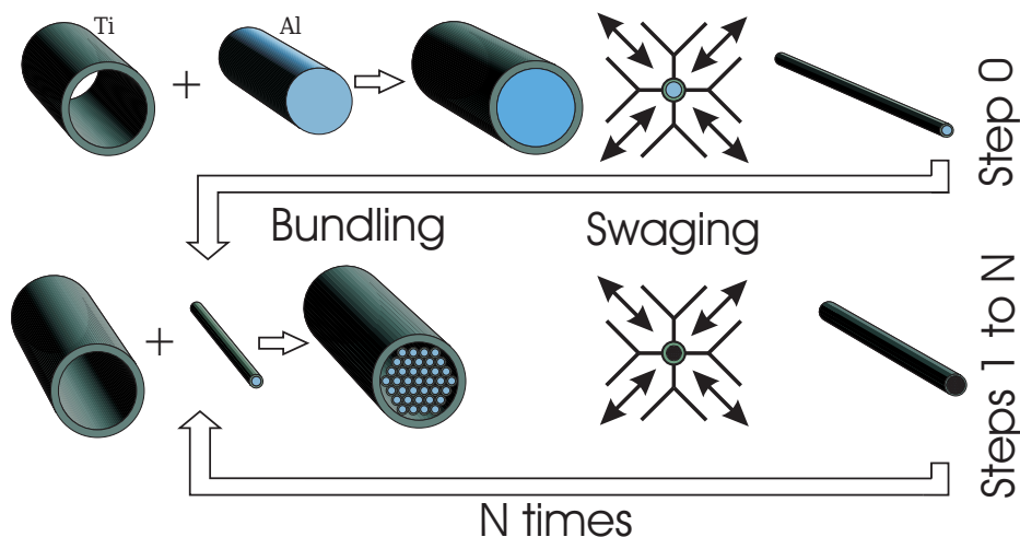
Abbildung 3.1: ASB Prozessschema; nach [5]
