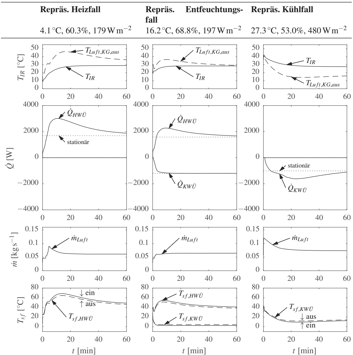
Abbildung A.8: Innenraumtemperatur T_{IR} , Heiz- und Kühlbedarfe \dot{Q}_{HWÜ} und \dot{Q}_{KWÜ} , Luftmassenstrom im Klimagerät \dot{m}_{KG} und sekundärfluidseitige Vor- und Rücklaufemperaturen für die repräsentativen Randbedingungen bei einer Konstantfahrt mit 50 km/h und einstündiger Konditionierung des Fahrzeugs.
