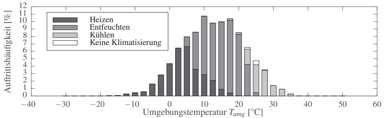
Abbildung 2.5: Auftrittshäufigkeit der Fälle Heizen, Kühlen und Entfeuchten gewichtet nach Bevölkerungsdichte und Tageszeit für Europa abhängig von T_{umg} .
