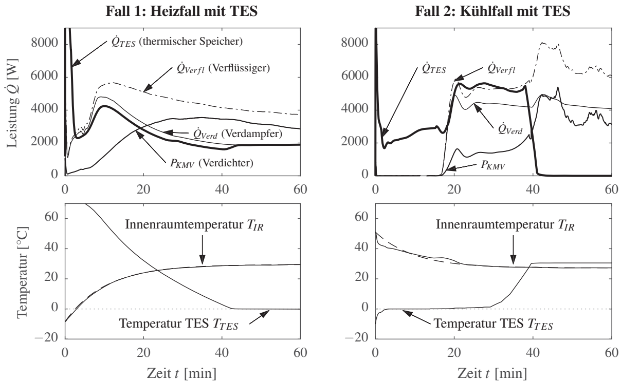
Abbildung 8.7: Simulationsergebnisse für einen Aufheizfall bei T_{umg} = -10^\circ\text{C} mit einem auf 90^\circ\text{C} vortempertierten TES und einen Abkühlfall bei T_{umg} = 35^\circ\text{C} , einer relativen Luftfeuchte von 37% und einer solaren Strahlung von 586\text{ W m}^{-1} nach einstündiger Konditionierung mit einem auf -10^\circ\text{C} vortempertierten TES.
