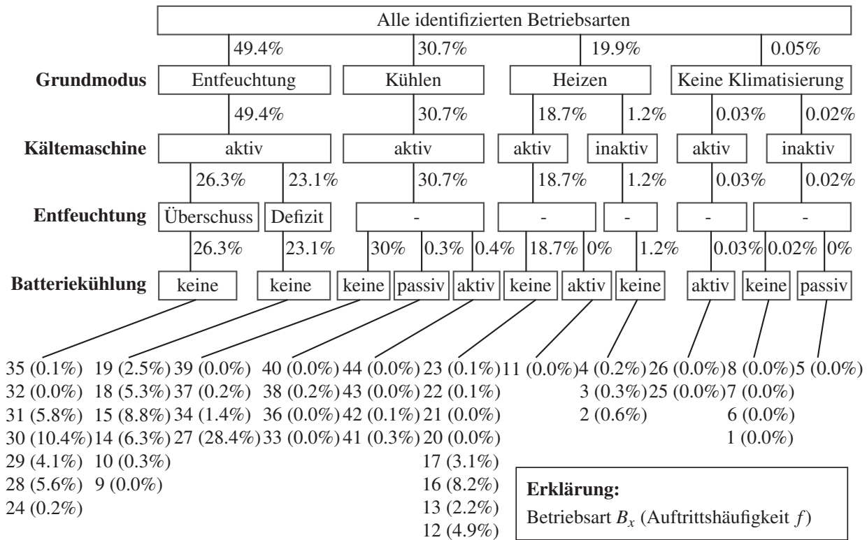
Abbildung 5.7: Klassifikation von Betriebsarten nach den Kriterien Grundmodus Innenraum, Kältemaschinen-/Wärmepumpenbetrieb, Entfeuchtungsbetrieb und Art der Batteriekühlung (ohne B_1 ).
