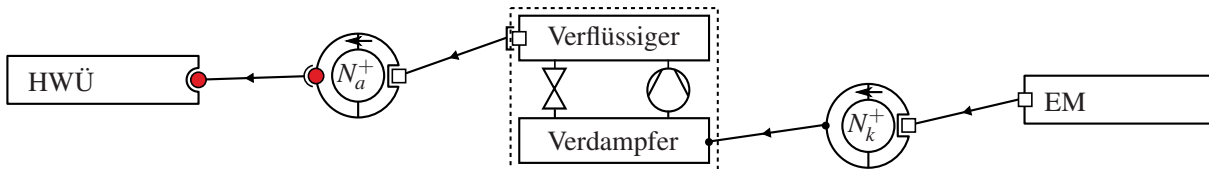
Abbildung 4.17: Zwei Betriebsarten für einen Hochlast-Kühlfall mit fünf aktiven Funktionen und für einen Wärmepumpen-Heizfall mit zwei aktiven Funktionen. Eine Betriebsart setzt sich aus mehreren Funktionen zusammen. Eine Funktion stellt über einen virtuellen Knoten eine Verbindung zwischen einer anfordernden und einer kompensierenden Systemkomponente her. Darstellungen von Betriebsarten werden automatisch generiert. Alle 44 auftretenden Betriebsarten befinden sich in Anhang E.
