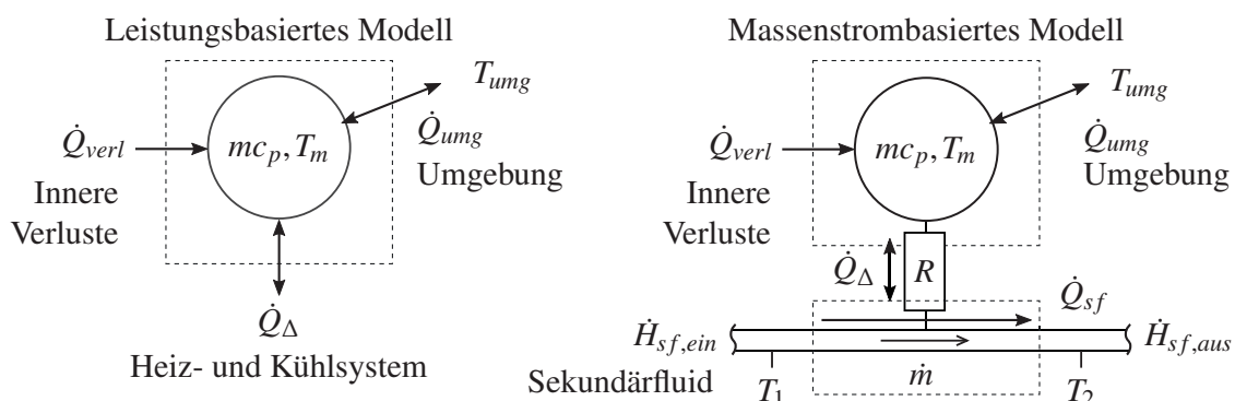
Abbildung 2.7: Thermische Punktmassenmodelle mit der repräsentativen Temperatur T_m und der thermischen Kapazität mc_p . Links: Die Leistung \dot{Q}_{\Delta} , die durch das Heiz- und Kühlsystem zu- oder abgeführt wird, ist vorgegeben. Rechts: Die Leistung \dot{Q}_{\Delta} , die durch das Heiz- und Kühlsystem zu- oder abgeführt wird, errechnet sich aus Temperatur und Massenstrom des Sekundärfluids und dem thermischen Widerstand R . Eine ausführliche Darstellung erfolgt in Anhang B.
