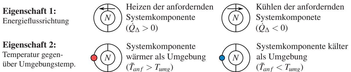
Abbildung 4.10: Die zwei grundlegenden Eigenschaften einer Heiz- oder Kühlanforderung ergeben sich aus Richtung des thermischen Energiestroms und Temperaturniveau der Systemkomponente relativ zur Umgebungstemperatur. Aus diesen zwei Eigenschaften folgen die Eigenschaften eines virtuellen Knotens.
