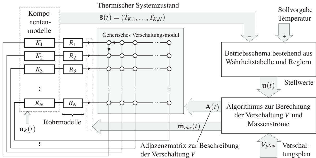
Abbildung 6.3: Übersicht des Simulationsmodells bestehend aus generischem Verschaltungsmodul für die Simulation des Sekundärkreislaufsystems und Betriebssystem zur Auswahl geeigneter Verschaltungen. Verschaltungen von Systemkomponenten ergeben sich aus den Pumpen- und Ventilstellwerten \mathbf{u} für einen gegebenen Verschaltungsplan.
