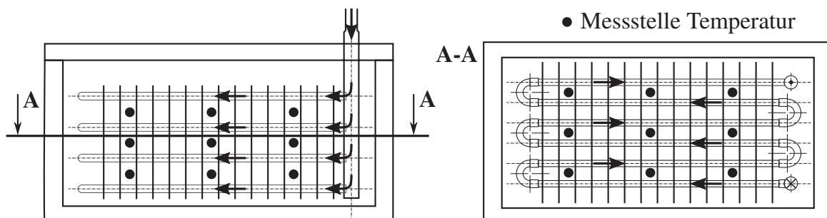
Abbildung 3.9: Schematischer Aufbau des thermischen Eis-Speichers für eine Speichermasse von 20 kg mit 27 Temperaturmessstellen.
