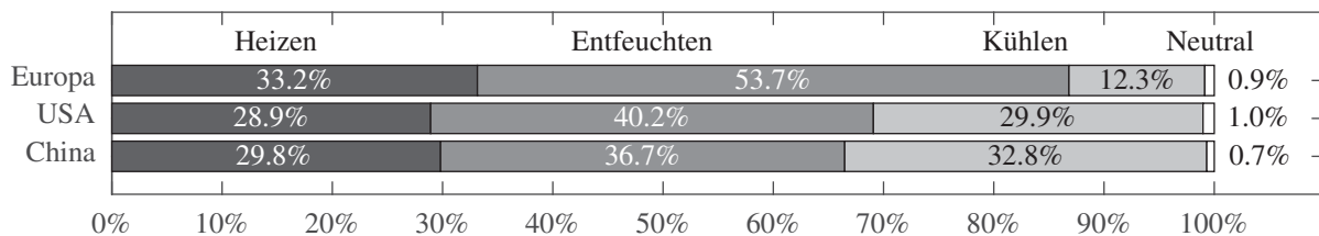
Abbildung 2.6: Auftrittshäufigkeit der Betriebsmodi Heizen, Entfeuchten und Kühlen.
