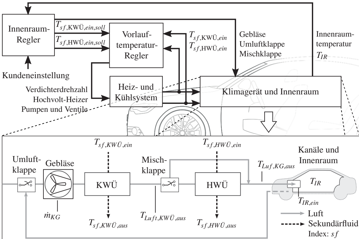
Abbildung 2.3: Schematische Übersicht des Klimatisierungssystems für das untersuchte Sekundärkreislaufsystem. Die ausführliche Darstellung erfolgt in Anhang A.
