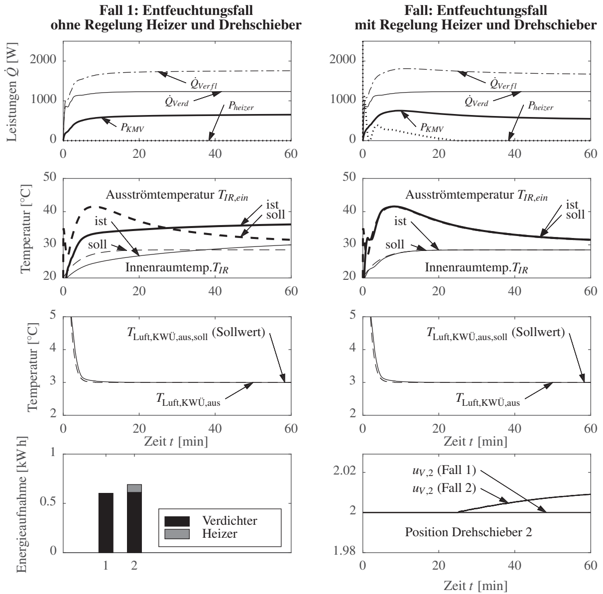
Abbildung 7.17: Vergleich des Entfeuchtungsberriebs ohne (links) und mit (rechts) Regelung des anfänglichen Defizits mit Hilfe des Heizers und späterem Überschuss mit Hilfe des Drehschiebers 2. Ohne Regelung von Heizer und Drehschieber 2 werden die Sollvorgaben für Ausströmtemperatur T_{IR,ein} und die Innenraumtemperatur T_{IR} nicht erreicht.
