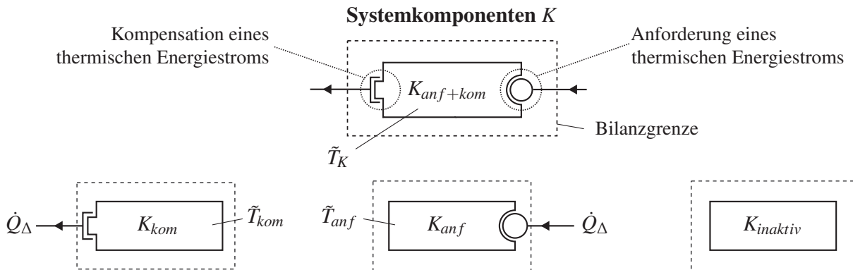
Abbildung 4.4: Vier Zustände, die eine Systemkomponente K annehmen kann: Anfordernd ( K_{anf} ), kompensierend ( K_{kom} ), beides ( K_{anf+kom} ) oder weder noch ( K_{inaktiv} ).
