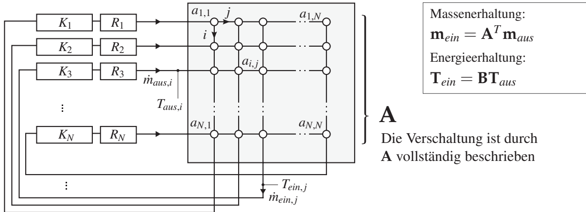
Abbildung 6.7: Generisches Verschaltungsmodul zur Beschreibung beliebiger Verschaltungen. Die Massenstrom-Abbildungs-Matrix \mathbf{A} kann als Adjazenzmatrix eines gerichteten Graphen, der genau die Verbindungen der einzelnen Komponenten zueinander beschreibt, interpretiert werden. Die Elemente der Matrix \mathbf{A} werden durch Knotenpunkte symbolisiert.
