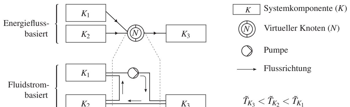
Abbildung 7.4: Eine mögliche Realisierung eines virtuellen Knotens N als Sekundärfluidkreislauf.
