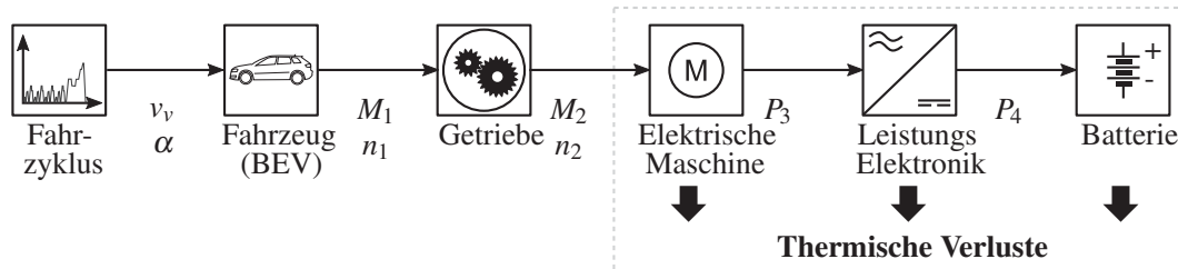
Abbildung B.3: Übersicht Antriebsstrangmodell
