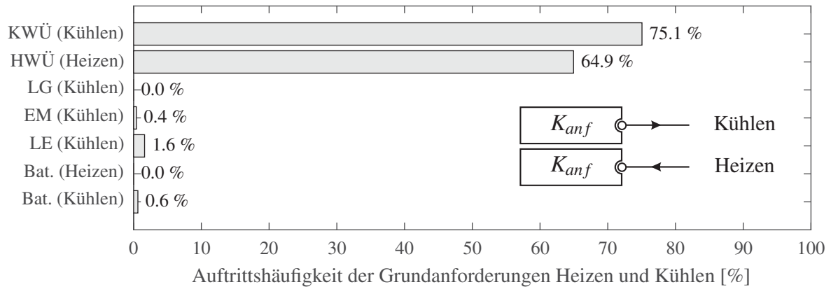
Abbildung 5.6: Auftrittshäufigkeiten der Anforderungen Heizen und Kühlen für alle anfordernden Systemkomponenten K_{anf} basierend auf 48 gewichteten Tagesfahrzyklen.
