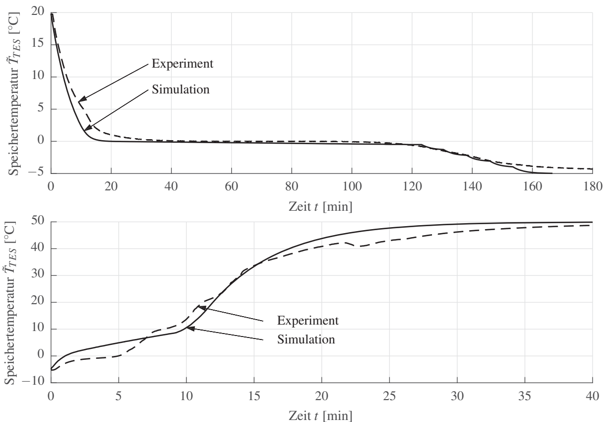
Abbildung 3.11: Gemittelte Speichertemperatur \tilde{T}_{TES} bei einem Beladevorgang (oben) und einem Entladevorgang (unten) eines thermischen Speichers mit einer Speichermasse von 20\text{ kg} und 15 Lamellen bei einem Sekundärfluidmassenstrom von \dot{m}_{sf} = 0.2\text{ kg s}^{-1} beziehungsweise \dot{m}_{sf} = 0.35\text{ kg s}^{-1} und einer Vorlauftemperatur von T_{sf, TES, ein} = -5^\circ\text{C} beim Beladen und T_{sf, TES, ein} = 50^\circ\text{C} beim Entladen.
