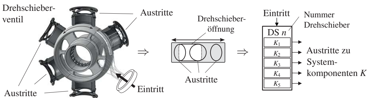
Abbildung 7.7: Aufbau eines Drehschieberventils zur Realisierung von Verschaltungsplänen durch kontinuierliche Verteilung von Fluidströmen auf mehrere mögliche Ausgänge.
