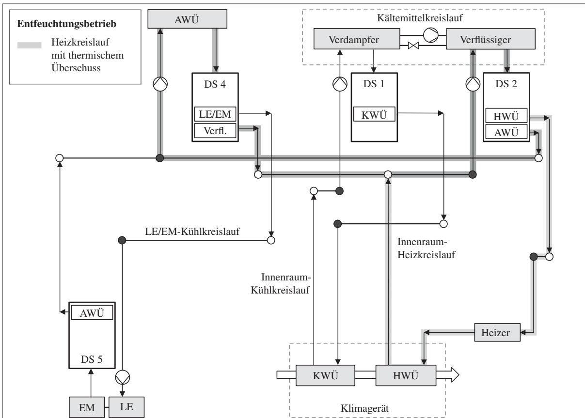
Abbildung 7.16: Verschaltung mit Entfeuchtungsbetrieb und gleichzeitiger Kühlung der Antriebskomponenten für den Verschaltungsplan aus Abbildung 7.9.
