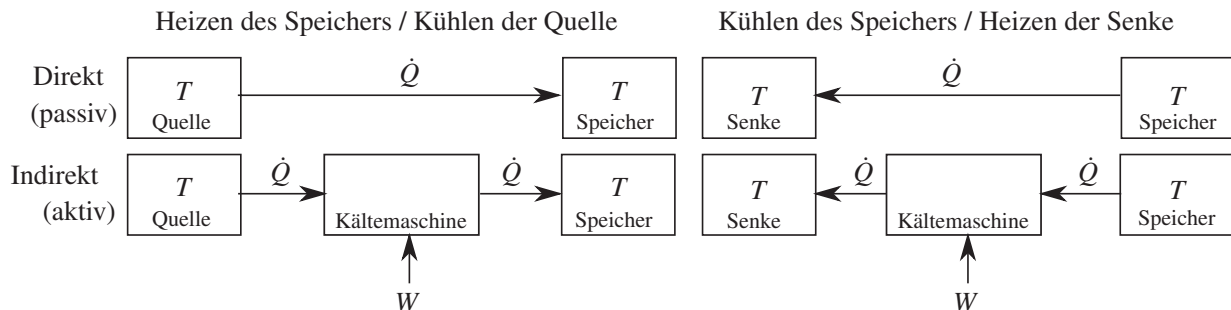
Abbildung 3.8: Direkte und indirekte Prozessführung des thermischen Speichers
