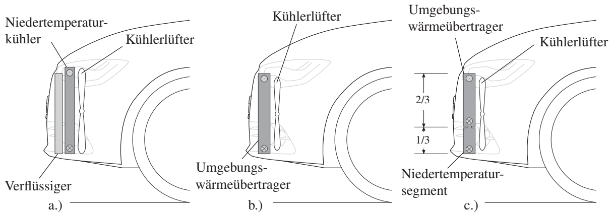
Abbildung 3.3: Kühlerpakete für ein konventionelles System (a), für ein sekundärkreislaufbasiertes System (b) sowie ein sekundärkreislaufbasiertes System mit Unterkühlungssegment zur Bereitstellung unterschiedlicher Temperaturniveaus (c). Legende: \odot = Zulauf Kühler, \otimes = Rücklauf Kühler.
