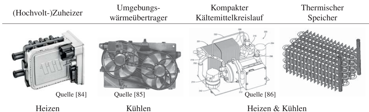
Abbildung 3.1: Systemkomponenten zur Bereitstellung von Heiz- und Kühlleistung.
