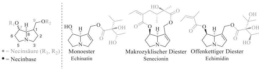
Abbildung 2-1: Basisstruktur der PAs (graue Markierung: Necinsäure, schwarze Markierung: Necinbase) sowie Strukturen der verschiedenen Estertypen am Beispiel von Echinatin (Monoester), Senecionin (makrozyklischer Diester) und Echimidin (offenkettiger Diester).
